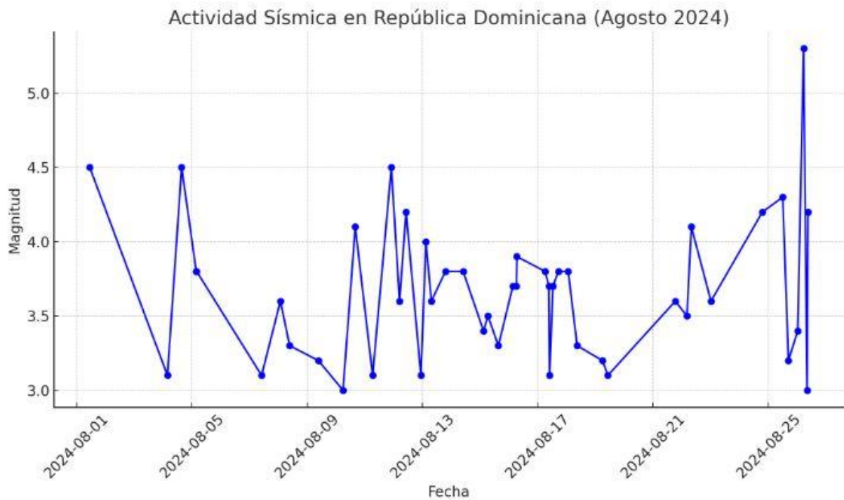
Ilustración 1: El gráfico muestra la magnitud de cada sismo registrado a lo largo del mes, lo que permite observar la variabilidad en la intensidad de los sismos en ese periodo.
